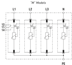
TNS (3Ph+N) - 4P
